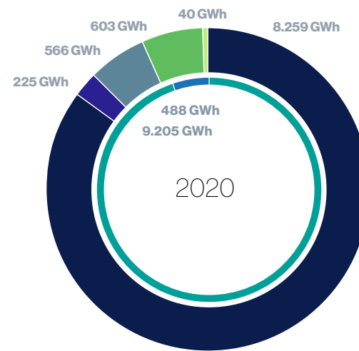
Gesamtenergieeinsatz 9.693 GWh
