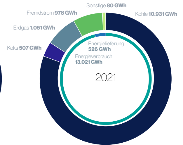
Gesamtenergieeinsatz 13.547 GWh
