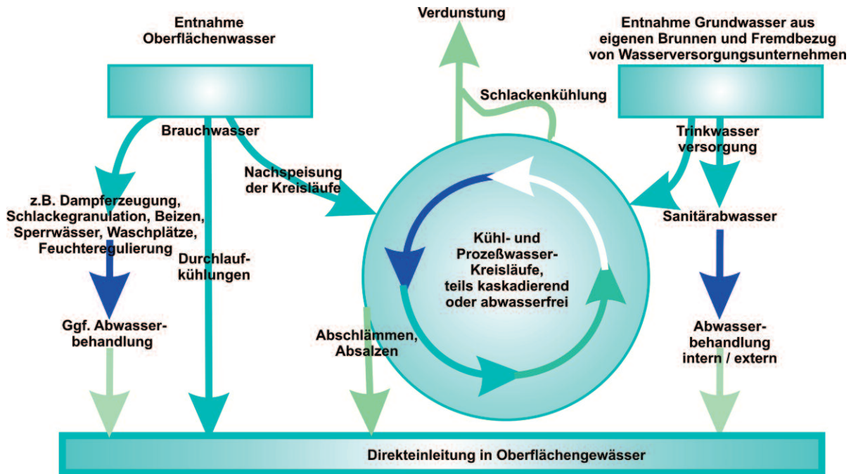
Gesamtübersicht Wasserkreislauf
